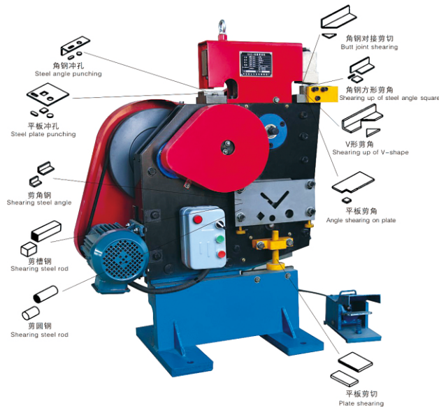
QA35-12冲剪机
