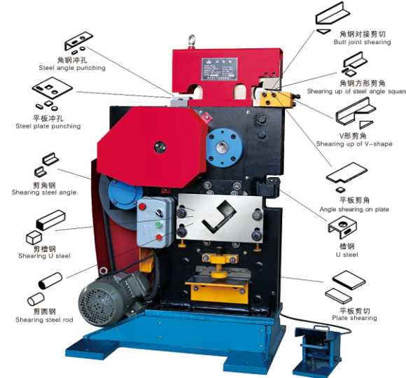
QA34-10角钢、槽钢冲剪机
