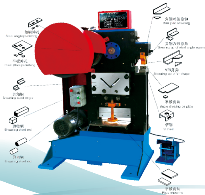
QA35-12冲剪机
